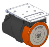
ezMCS/L/160/+ Federung light mit 3 Federn
