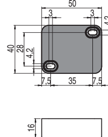
Actionneur SM E•T
