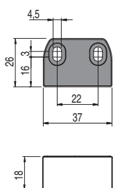
Actionneur SM G•T
