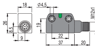
Capteur ST G••••MP avec connecteur M12
