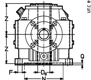
Modello - Type albero lento cavo - hollow low speed shaft FO4 ... ( i \leq 2 )
