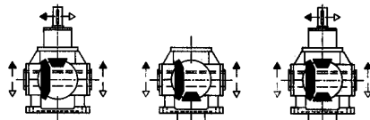
Modello - Type albero lento cavo - hollow low speed shaft PO4 ... ( i \leq 2 )
