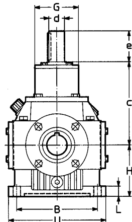
Modello - Type albero lento cavo - hollow low speed shaft PO4 ... ( i \leq 2 )
