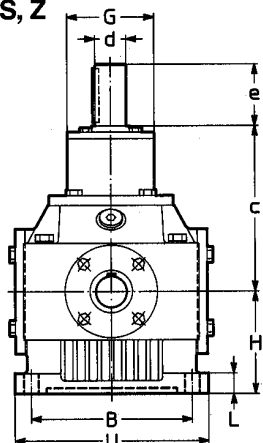
Modello - Type normale - standard PO1 ... (80 ... 200), PO2 ... (250, 320, i \geq 2,5 ) albero lento maggiorato - oversized low speed shaft PO3 ... ( i \leq 2 )
